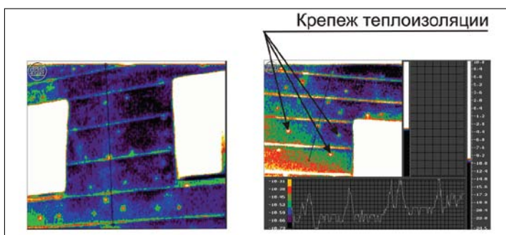
Термограммы утепленных фасадов (теплоизоляция закреплена дюбелями со стальным РЭ)
